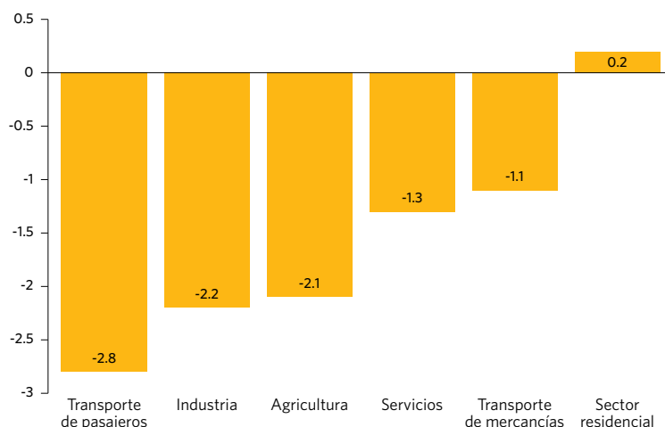
Tasa de crecimiento anual combinada de la intensidad energética final en los sectores de usuarios finales, 2012-2014 (porcentaje)
